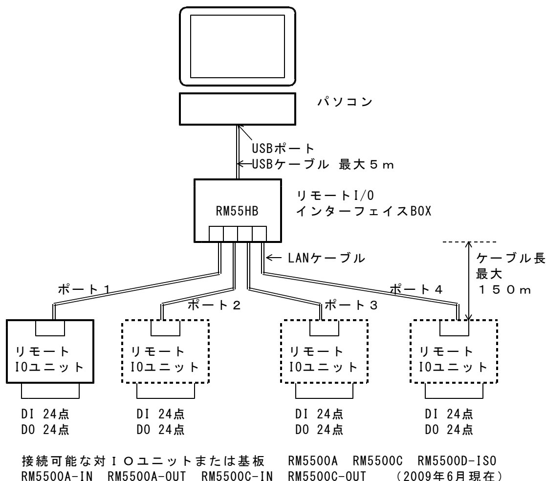
【図1. 1】 RM5500リモート I/Oシステム接続概要
