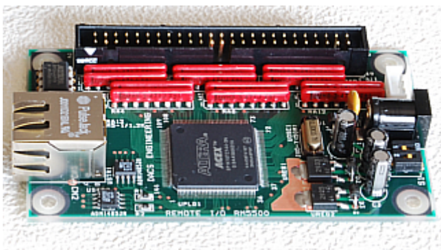
リモートIO基板 PWM 24chパルス出力 RM5500A-RCP24
