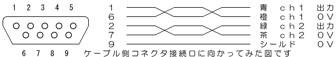
9DS-500 標準ケーブル長 50cm
