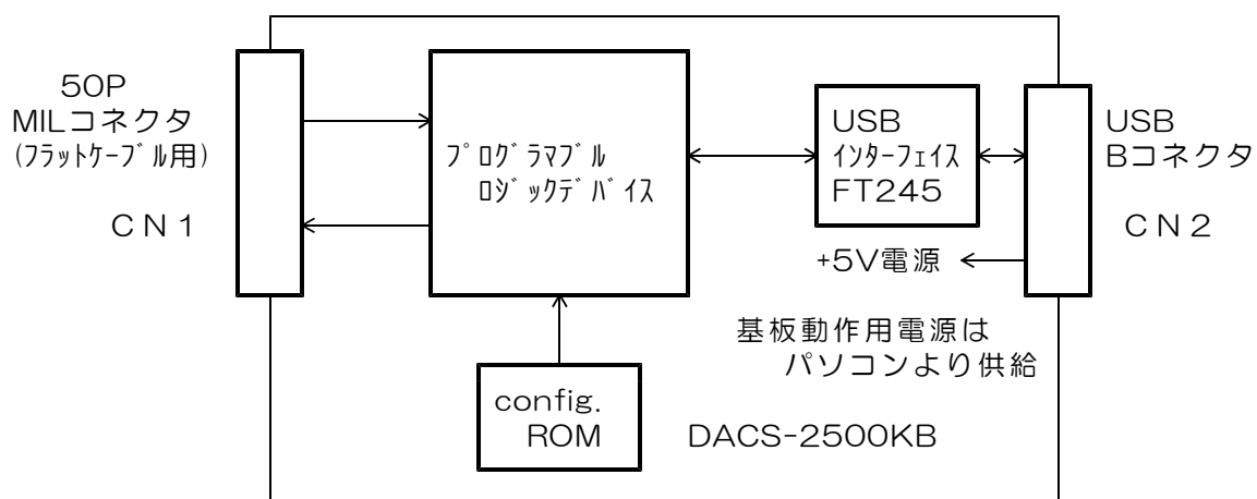
図1. 1 DACS-2500KB-SCN3/CNT3 ブロック図
