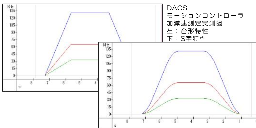
図14. 2 自動リピートモードでの周波数変化測定例
