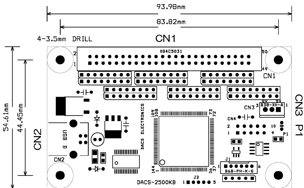
図1. 2 DACS-2500KB-SCN3/CNT3 外形図
