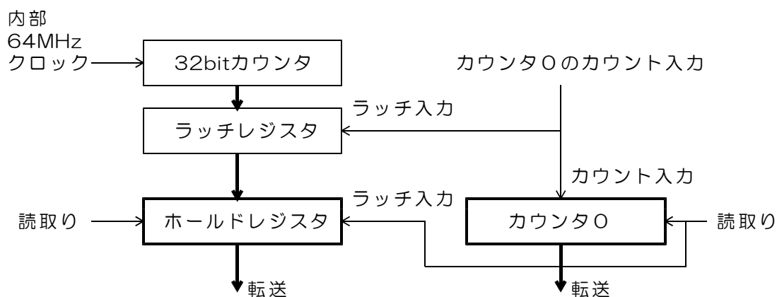
図14. 1 自動リピートモードでのホールドレジスタ
