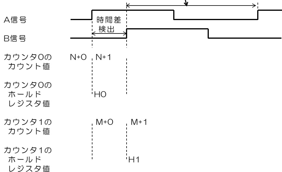
図14. 3 自動リピートモードでの2信号の時間差検出
