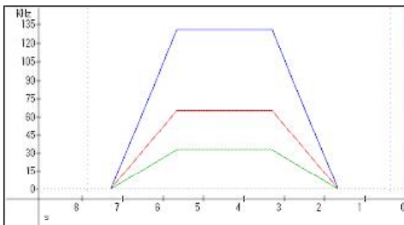
【図2.3】 台形加減速とS字加減速の実測例（カウンタDACS-2500KB-SCN3使用）
